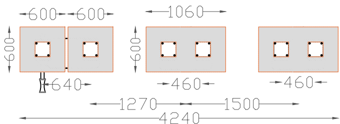
PLANTA . ESQUEMA DE FIXAÇÃO PLAN . INSTALLATION PLAN
