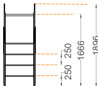
ALÇADO FRONTAL FRONT VIEW
