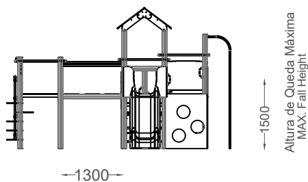
ALÇADO FRONTAL FRONT VIEW
