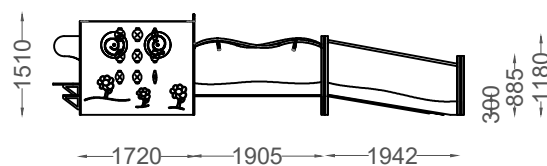
ALÇADO FRONTAL FRONT VIEW
