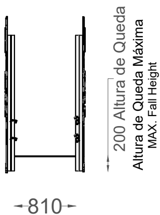
ALÇADO LATERAL SIDE VIEW
