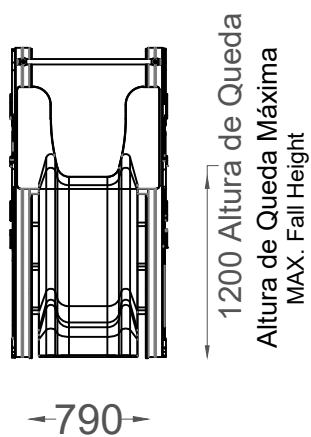
ALÇADO LATERAL SIDE VIEW
