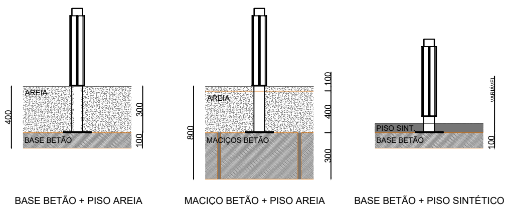
BASE BETÃO + PISO AREIA
