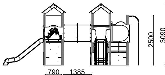
ALÇADO FRONTAL FRONT VIEW
