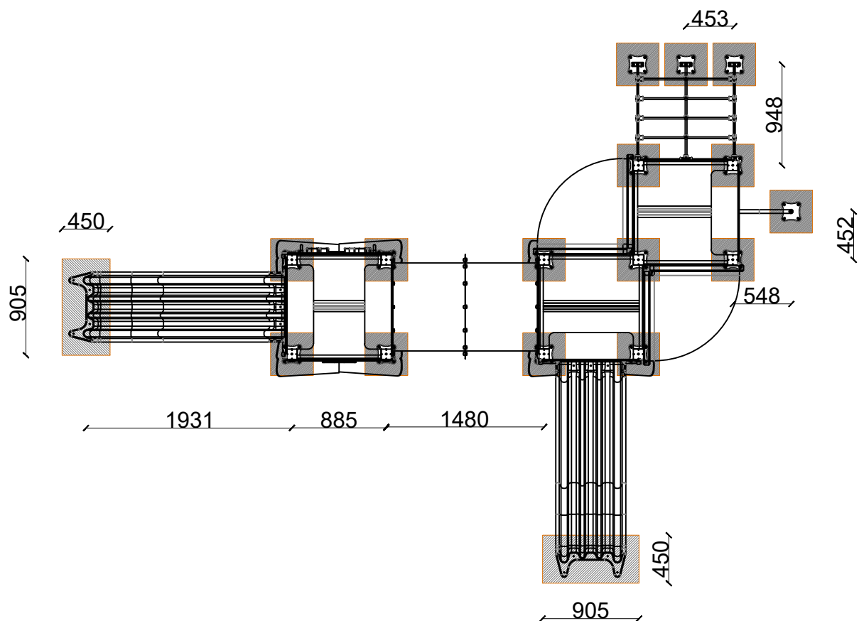
PLANTA . ESQUEMA DE FIXAÇÃO PLAN . INSTALLATION PLAN
