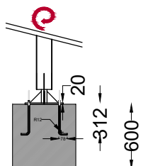
ALÇADO
