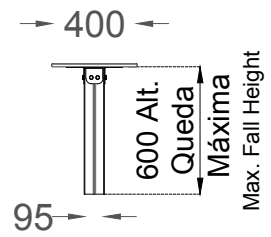
ALÇADO LATERAL SIDE VIEW
