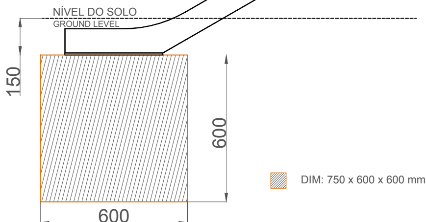
ALÇADO LATERAL . ESQUEMA DE FIXAÇÃO SIDE VIEW . INSTALLATION PLAN
