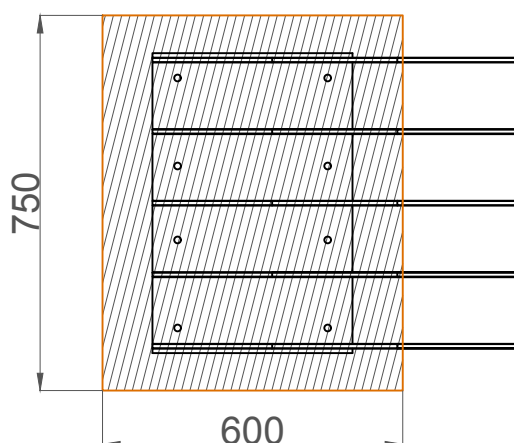
PLANTA . ESQUEMA DE FIXAÇÃO PLAN . INSTALLATION PLAN
