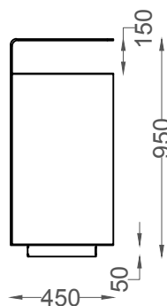
ALÇADO LATERAL SIDE VIEW
