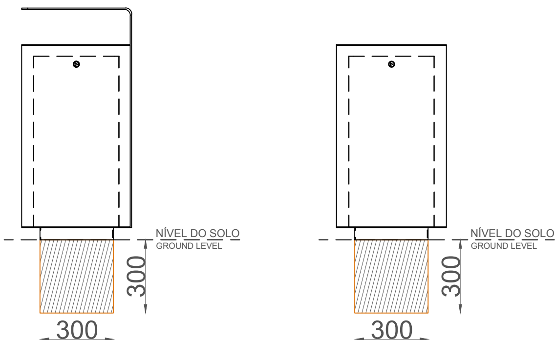
ALÇADO POSTERIOR . ESQUEMA DE FIXAÇÃO REAR VIEW . INSTALLATION PLAN
