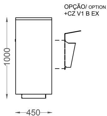
ALÇADO POSTERIOR REAR VIEW
