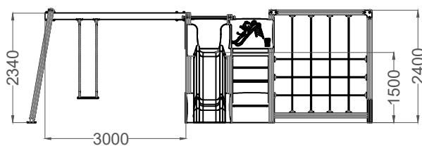
ALÇADO FRONTAL FRONT VIEW
