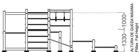
ALÇADO FRONTAL FRONT VIEW
