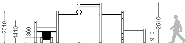
ALÇADO LATERAL SIDE VIEW
