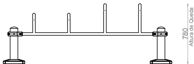
ALÇADO - INDICAÇÃO DA ALTURA DE QUEDA
