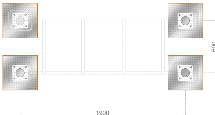
PLANTA - ESQUEMA DE MACIÇOS
