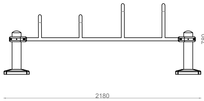
ALÇADO FRONTAL
