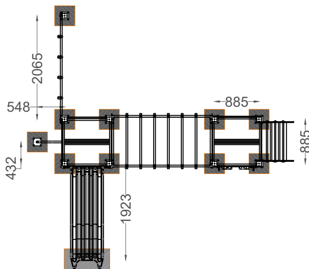
PLANTA . ESQUEMA DE FIXAÇÃO PLAN . INSTALLATION PLAN
