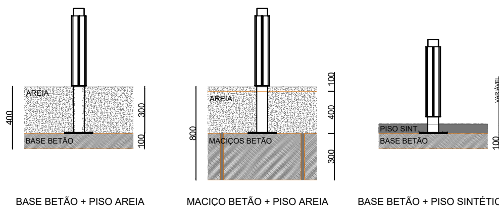
BASE BETÃO + PISO AREIA
