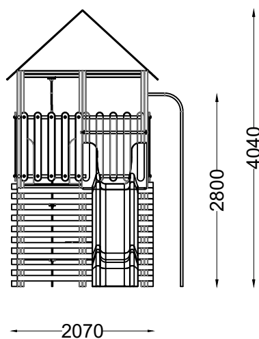
ALÇADO FRONTAL FRONT VIEW
