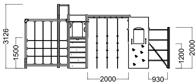
ALÇADO FRONTAL FRONT VIEW
