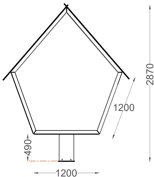
ALÇADO FRONTAL FRONT VIEW
