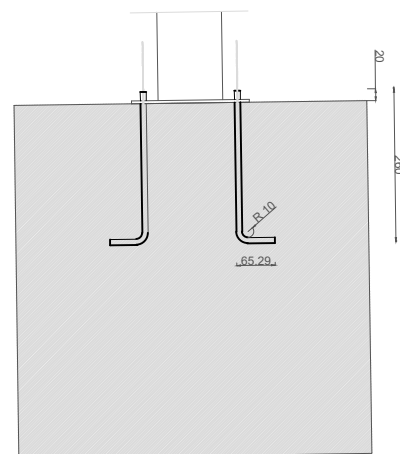
ALÇADO
