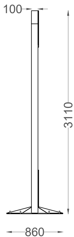
ALÇADO LATERAL SIDE VIEW
