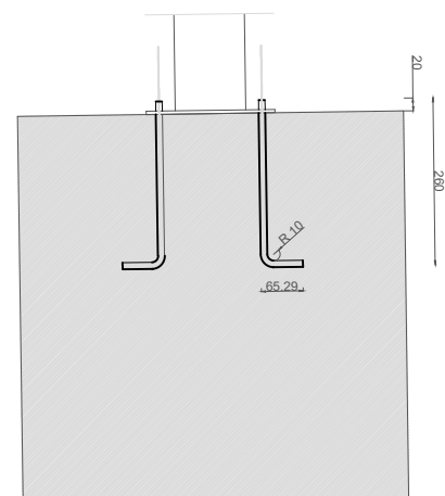
ALÇADO
