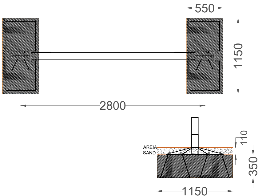
PLANTA . ESQUEMA DE FIXAÇÃO PLAN . INSTALLATION PLAN
