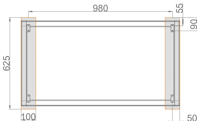
PLANTA . ESQUEMA DE MACIÇOS
