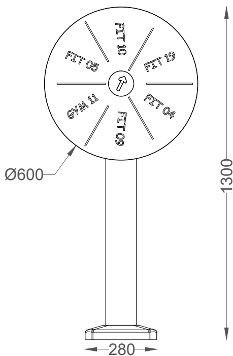
ALÇADO FRONTAL FRONT VIEW
