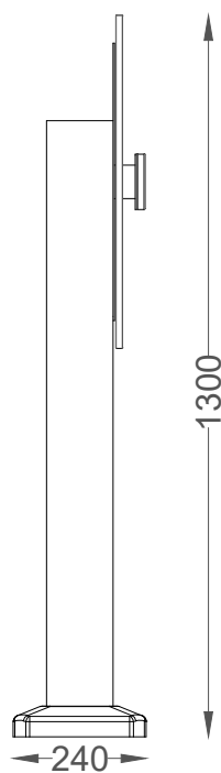
ALÇADO LATERAL SIDE VIEW
