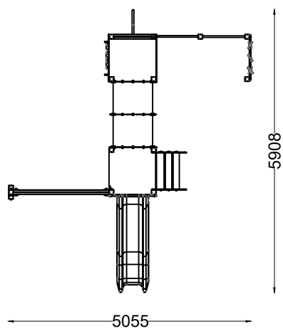
PLANTA PLAN
