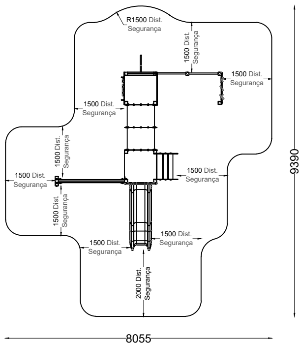
PLANTA - ESPAÇO DE SEGURANÇA NECESSÁRIO PLAN - SAFETY SPACE REQUIRED
