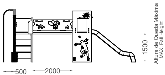
ALÇADO LATERAL SIDE VIEW
