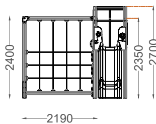
ALÇADO FRONTAL FRONT VIEW
