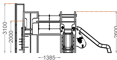
ALÇADO LATERAL SIDE VIEW
