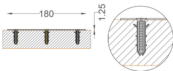
ALÇADO LATERAL . FIXAÇÃO EM BUCHA PLÁSTICA SIDE VIEW . Screws in plastic fixing
