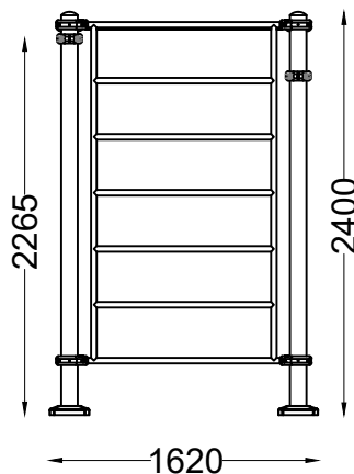
ALÇADO FRONTAL FRONT VIEW
