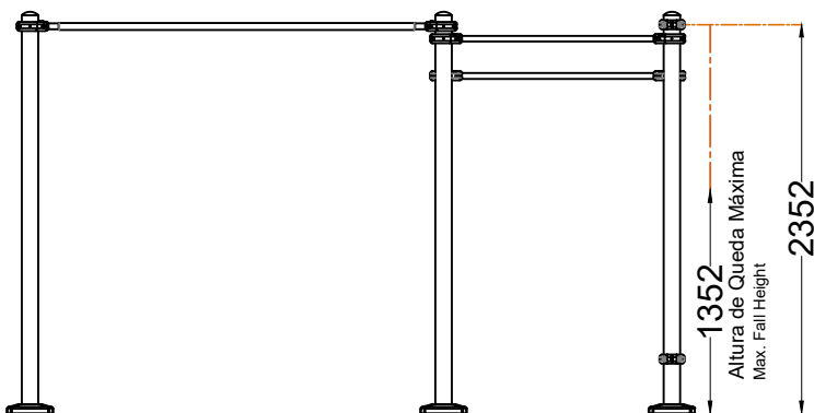
ALÇADO LATERAL SIDE VIEW
