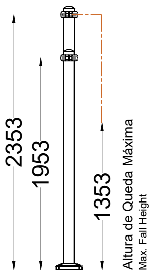
ALÇADO LATERAL SIDE VIEW
