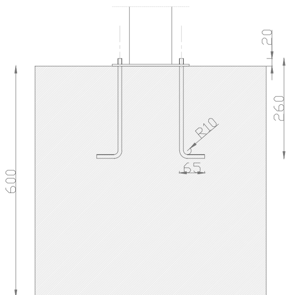
ALÇADO
