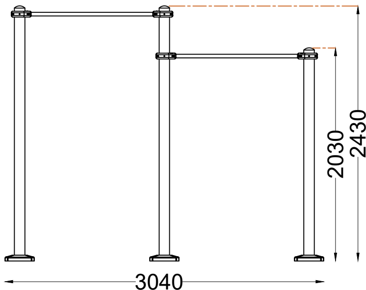
ALÇADO FRONTAL FRONT VIEW
