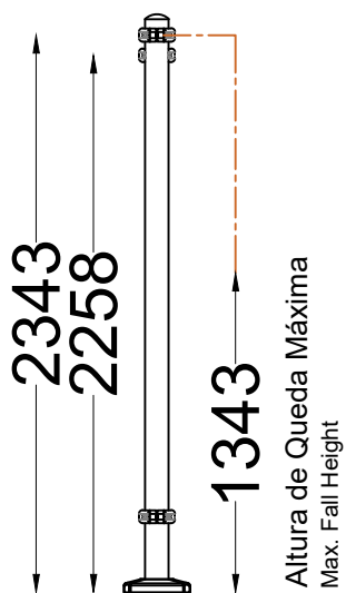
ALÇADO LATERAL SIDE VIEW
