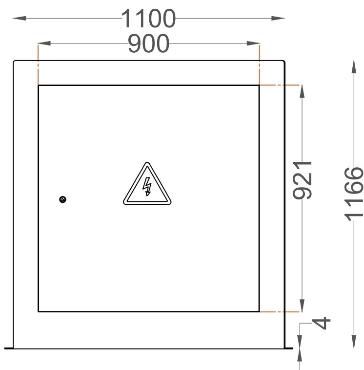
ALÇADO FRONTAL FRONT VIEW
