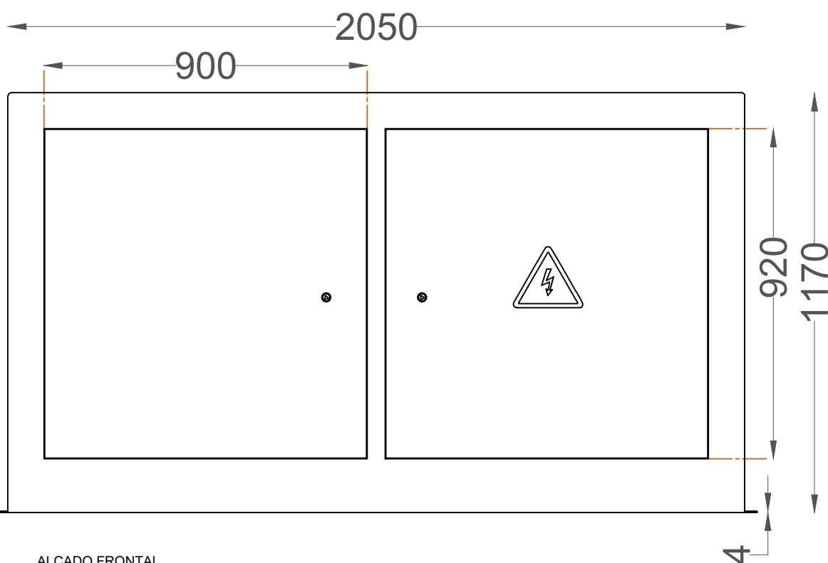
ALÇADO FRONTAL FRONT VIEW
