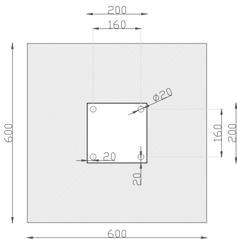
PLANTA
