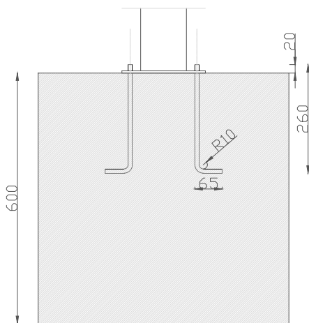
ALÇADO
