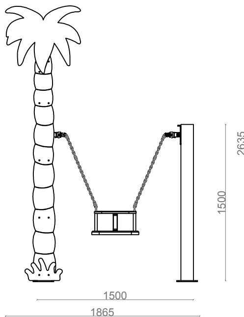
ALÇADO FRONTAL
