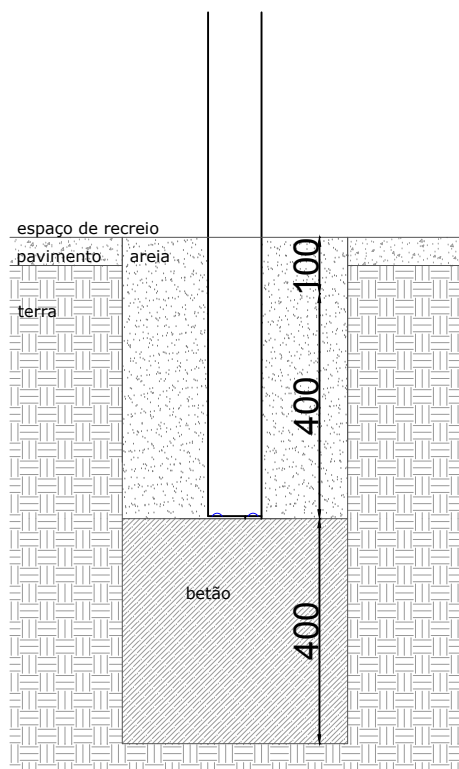
ESQUEMA DE FIXAÇÃO POR ENTERRAMENTO
