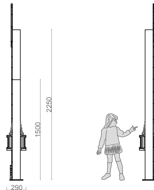
ALÇADO LATERAL
