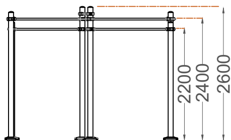
ALÇADO FRONTAL FRONT VIEW
