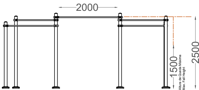
ALÇADO LATERAL SIDE VIEW
