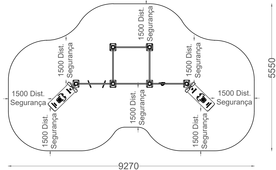
PLANTA - ESPAÇO DE SEGURANÇA NECESSÁRIO PLAN - SAFETY SPACE REQUIRED
