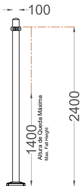
ALÇADO LATERAL SIDE VIEW
