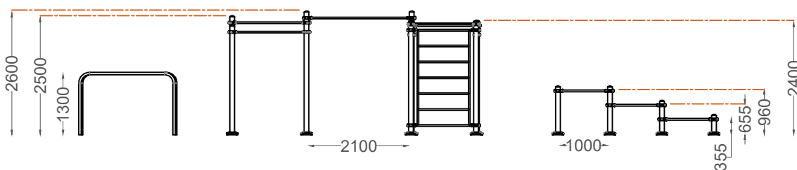
ALÇADO LATERAL SIDE VIEW
