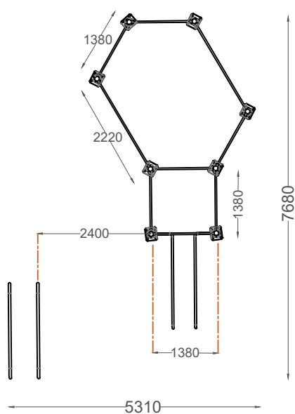
PLANTA - ESPAÇO DE SEGURANÇA NECESSÁRIO PLAN - SAFETY SPACE REQUIRED
