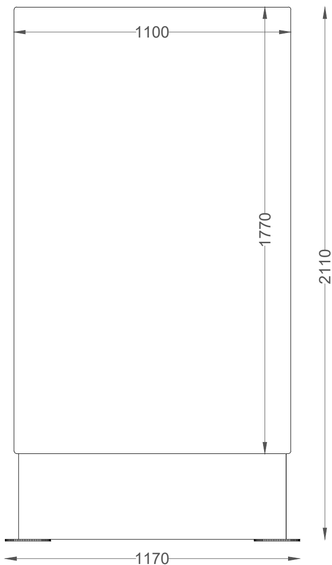
ALÇADO FRONTAL FRONT VIEW
