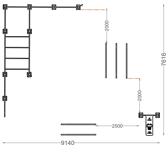
PLANTA PLAN
