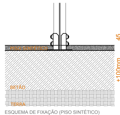
ESQUEMA DE FIXAÇÃO (PISO SINTÉTICO)
