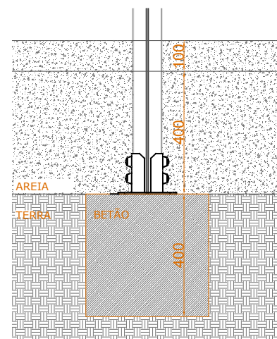
ESQUEMA DE FIXAÇÃO (PISO DE AREIA)
