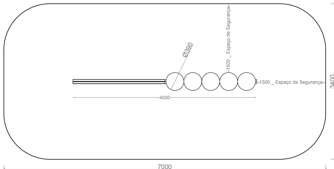
PLANTA _ ENQUADRAMENTO DO EQUIPAMENTO NO ESPAÇO DE SEGURANÇA NECESSÁRIO
