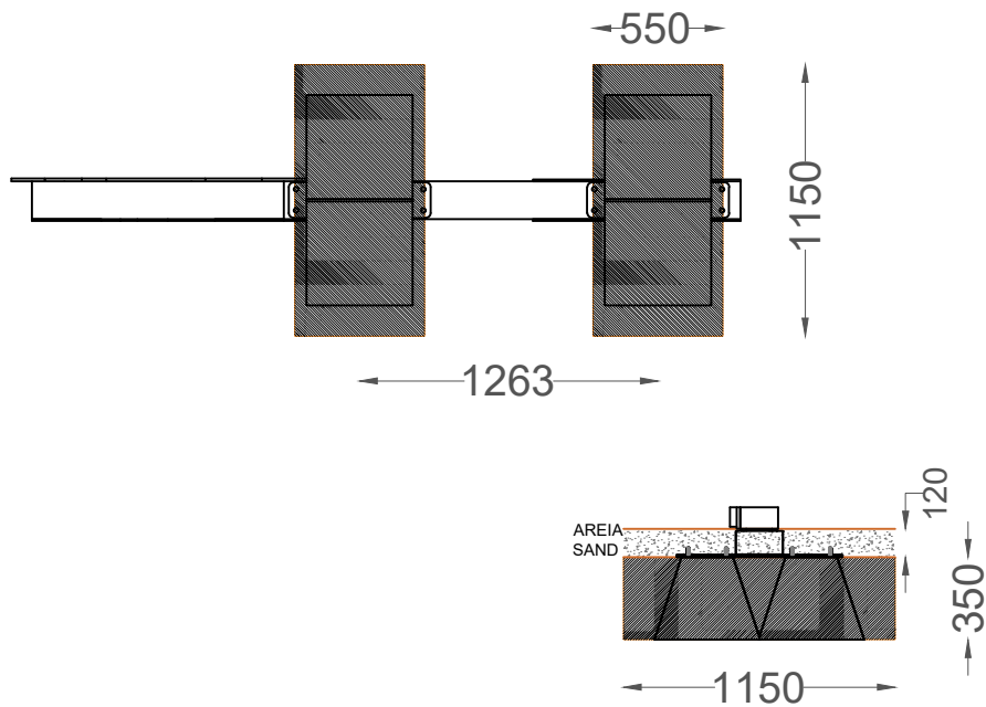
PLANTA . ESQUEMA DE FIXAÇÃO PLAN . INSTALLATION PLAN
