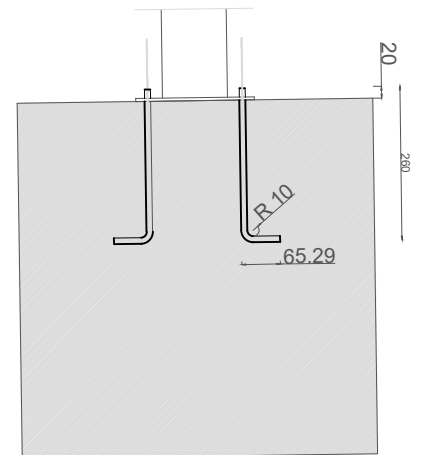
ALÇADO
