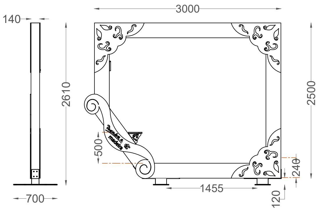
ALÇADO LATERAL SIDE VIEW
