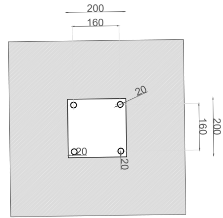
PLANTA
