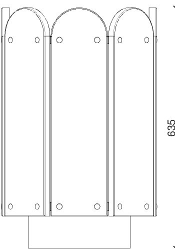
ALÇADO
