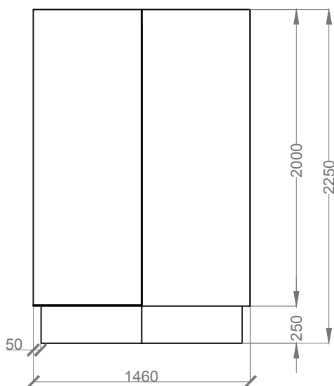
ALÇADO FRONTAL
