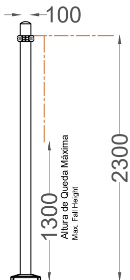
ALÇADO LATERAL SIDE VIEW
