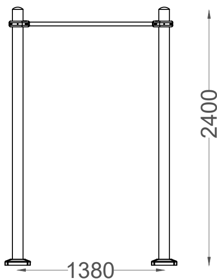
ALÇADO FRONTAL FRONT VIEW
