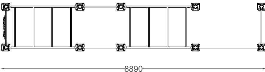
PLANTA PLAN
