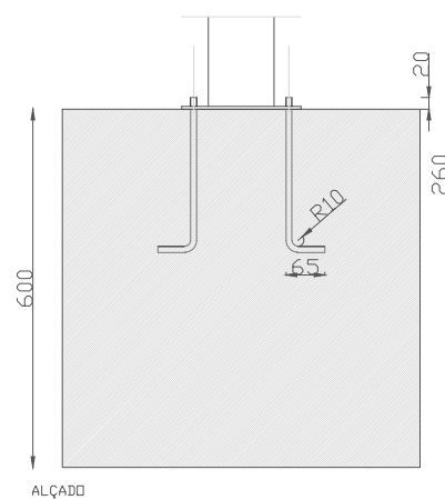
ALÇADO
