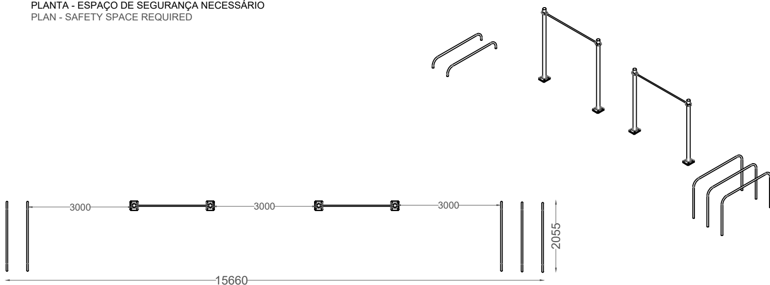
PLANTA PLAN
