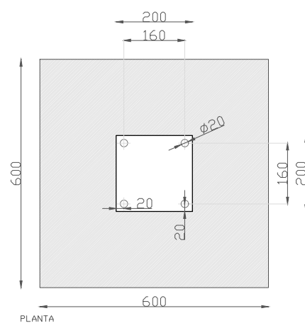
PLANTA
