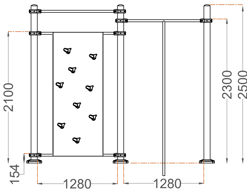
ALÇADO FRONTAL FRONT VIEW
