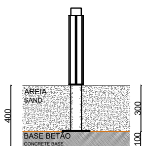
BASE BETÃO + PISO AREIA CONCRETE BASE + SAND LAYER
