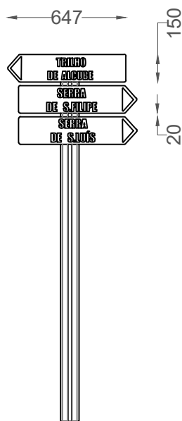
ALÇADO FRONTAL FRONT VIEW
