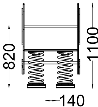
ALÇADO FRONTAL FRONT VIEW
