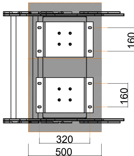
PLANTA, Esquema de Fixação
